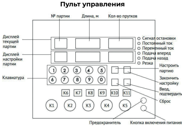
Рисунок 3. Пульт управления
