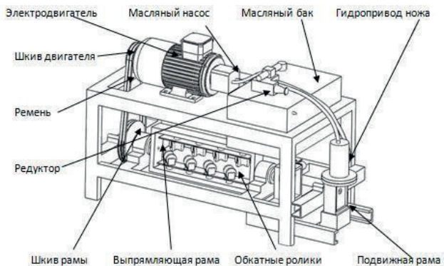
Рисунок 1. Устройство станка
