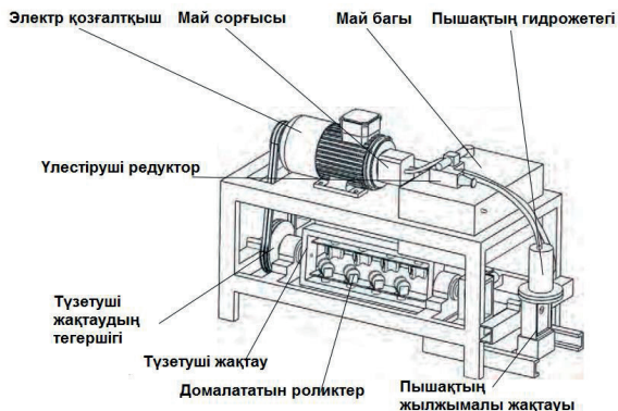
Сурет 1. Станоктың құрылымы
