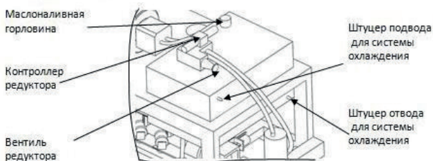
Рисунок 2. Устройство гидросистемы
