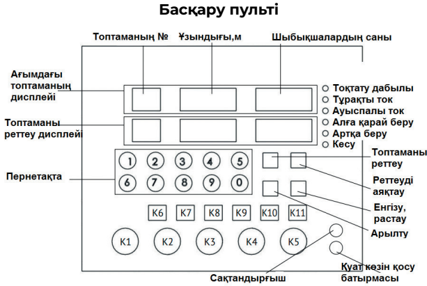
Сурет 3. Басқару пульті
