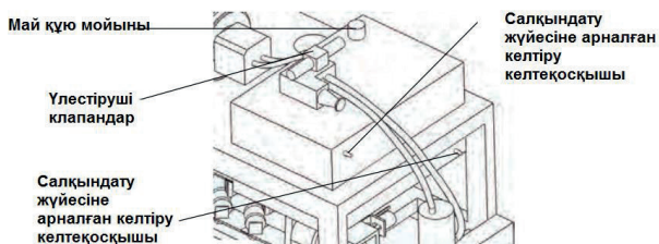
Сурет 2. Гидрожүйенің құрылымы
